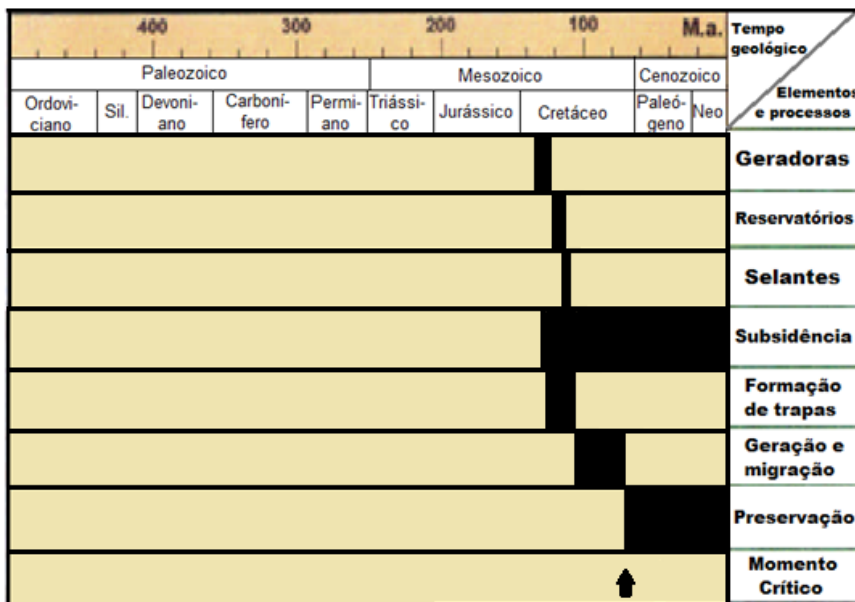
Figura 18: Carta de eventos do sistema petrolífero Codó-Tutóia (!).
