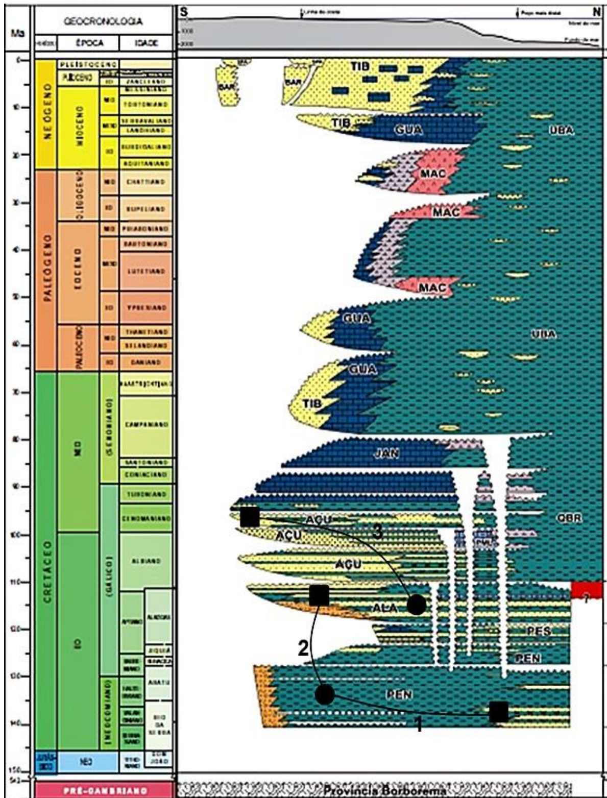
Figura 23: Sistemas petrolíferos da bacia Potiguar: 1: Pendência-Pendência (!), 2: Pendência-Alagamar (!), 3: Alagamar-Açu (!).
