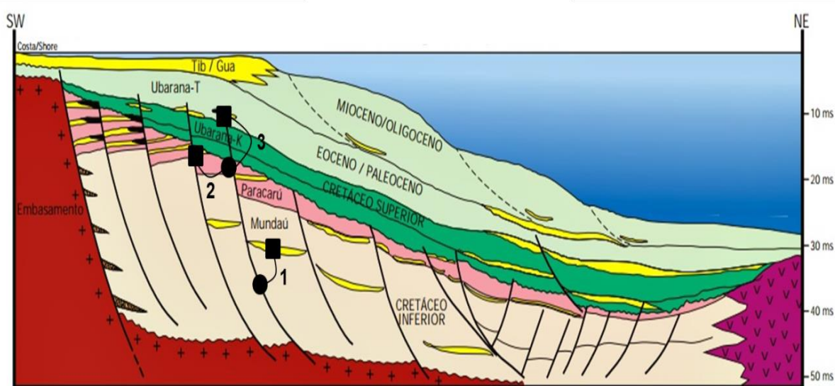
Figura 21: Seção geológica e seus respectivos sistemas petrolíferos: 1) Mundaú-Mundaú (!), 2) Paracuru-Paracuru (!) e 3) Paracuru-Ubarana (!).
