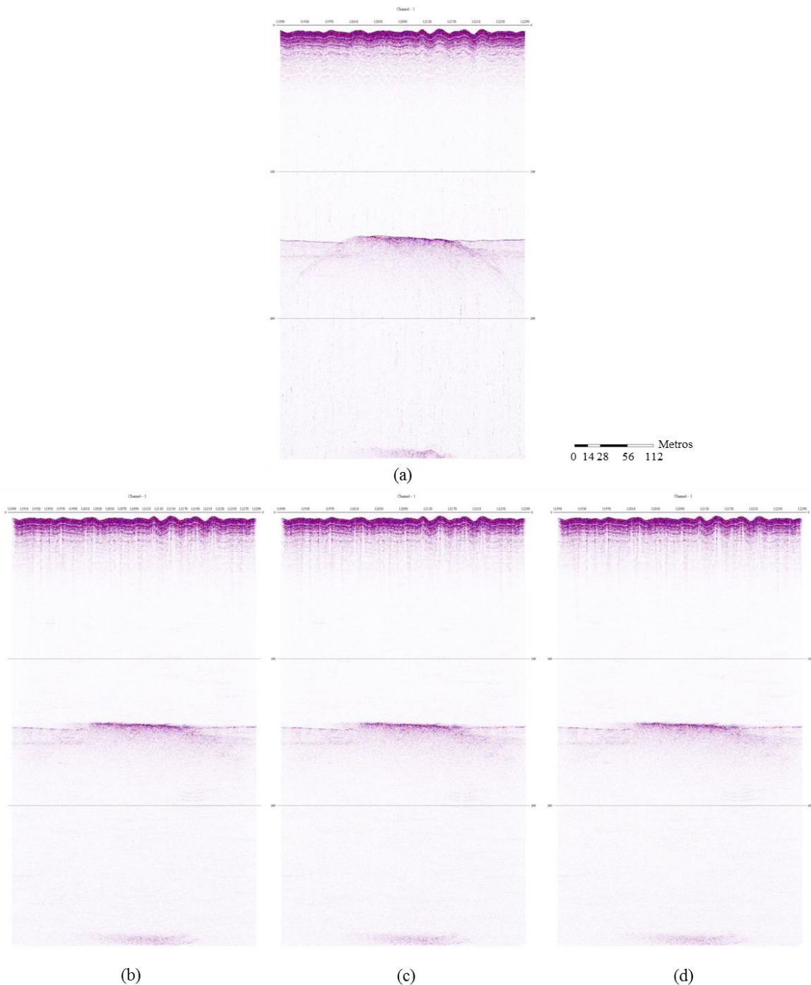
Figura 24: Seções sísmicas referentes ao (a) registro pré-migrado e a cada um dos três testes com diferentes velocidades para a etapa de migração, sendo utilizado em (b) 1450 m/s, em (c) 1500 m/s e em (d) 1550 m/s.
