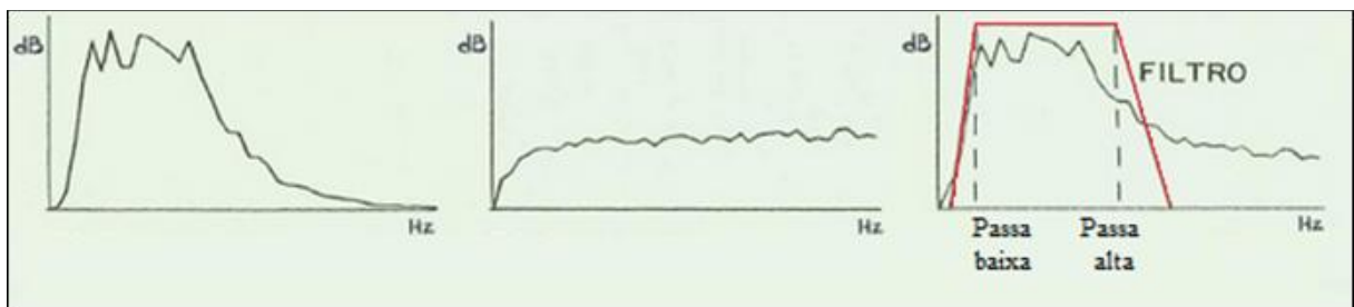
Figura 4: Espectros de amplitude x frequência referentes: em (a) apenas ao sinal sísmico; (b) apenas ao ruído; e em (c) ao dado sísmico como um todo (sinal e ruído), exemplificando o formato de um filtro do tipo passa-banda e indicando os parâmetros que devem ser utilizados para a filtragem.
