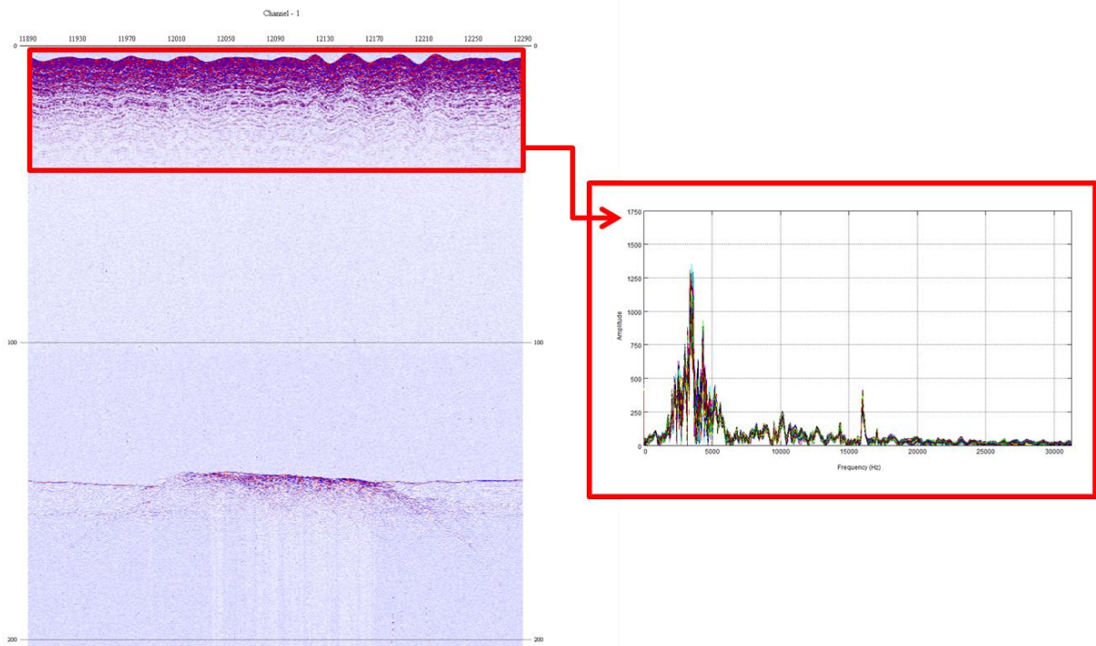
Figura 16: Destaque (vermelho) do ruído associado a onda direta e seu respectivo espectro de amplitude x frequência, calculado apenas para a região em destaque. Observa-se uma distribuição bastante similar com o espectro referente as reflexões principais.
