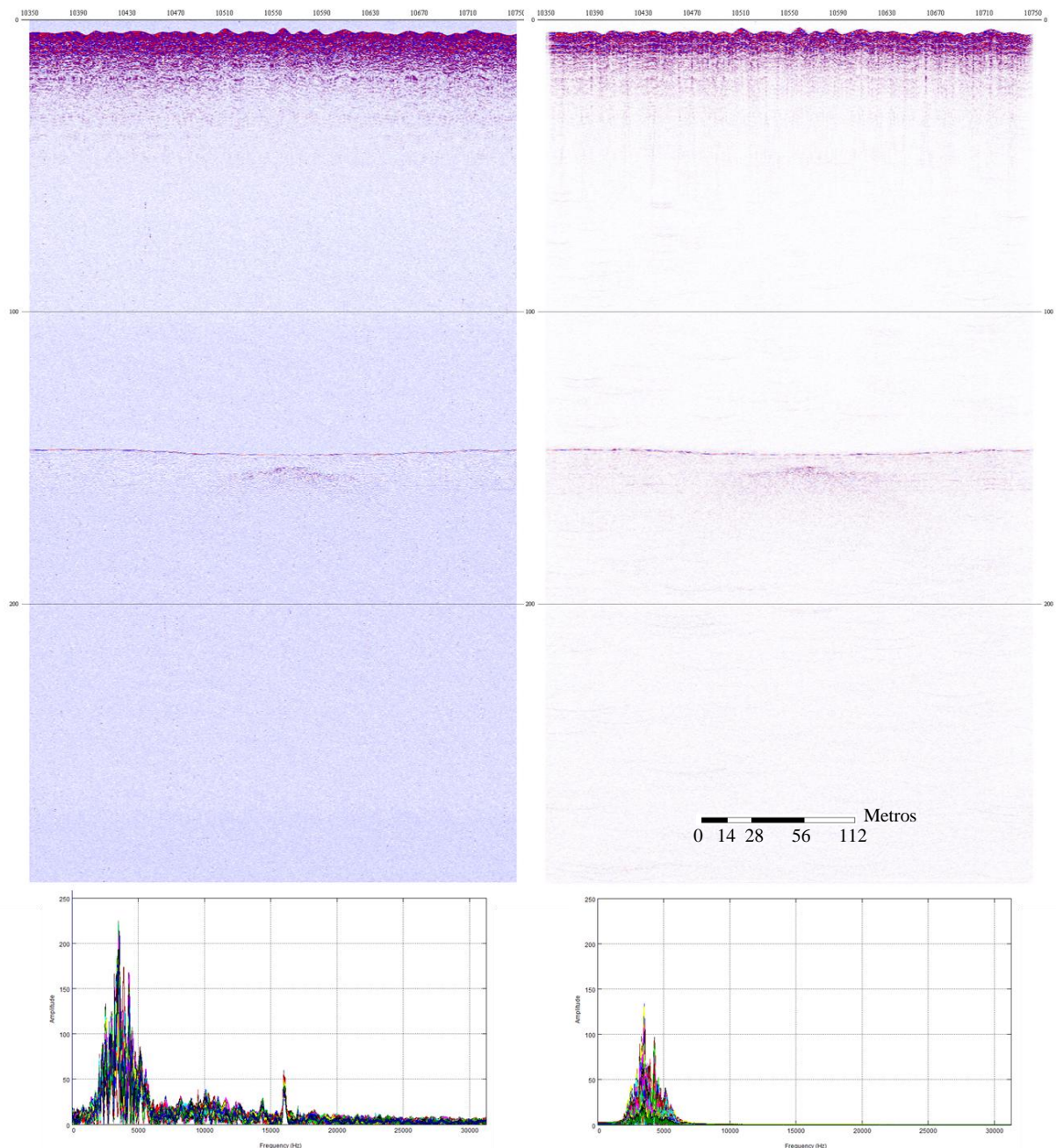
Figura 26: Seções sísmicas referentes a linha “FEC_22”, sendo em (a) o dado bruto e em (b) a seção pós-processada.
