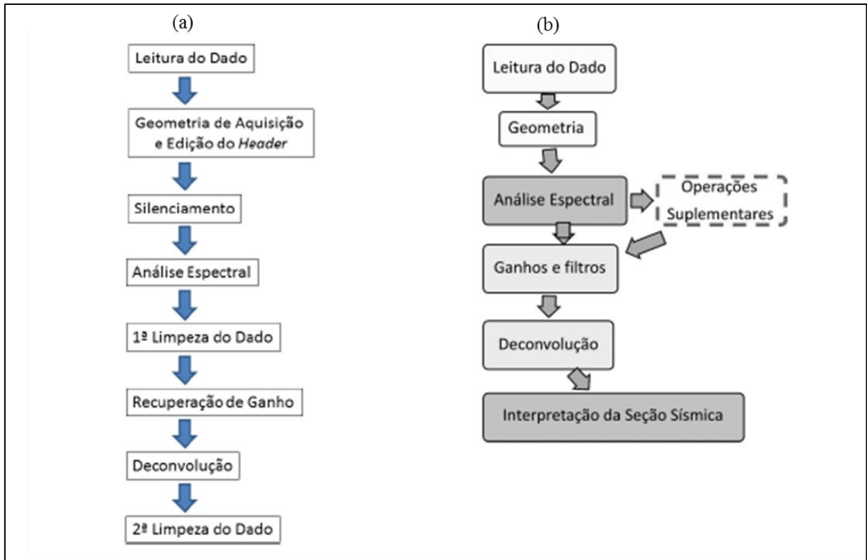
Figura 10: Fluxogramas de processamento sísmico associado a dados de alta resolução adquiridos através de equipamentos monocal. (a) Marino et al., 2012; (b) Gomes et al., 2010.
